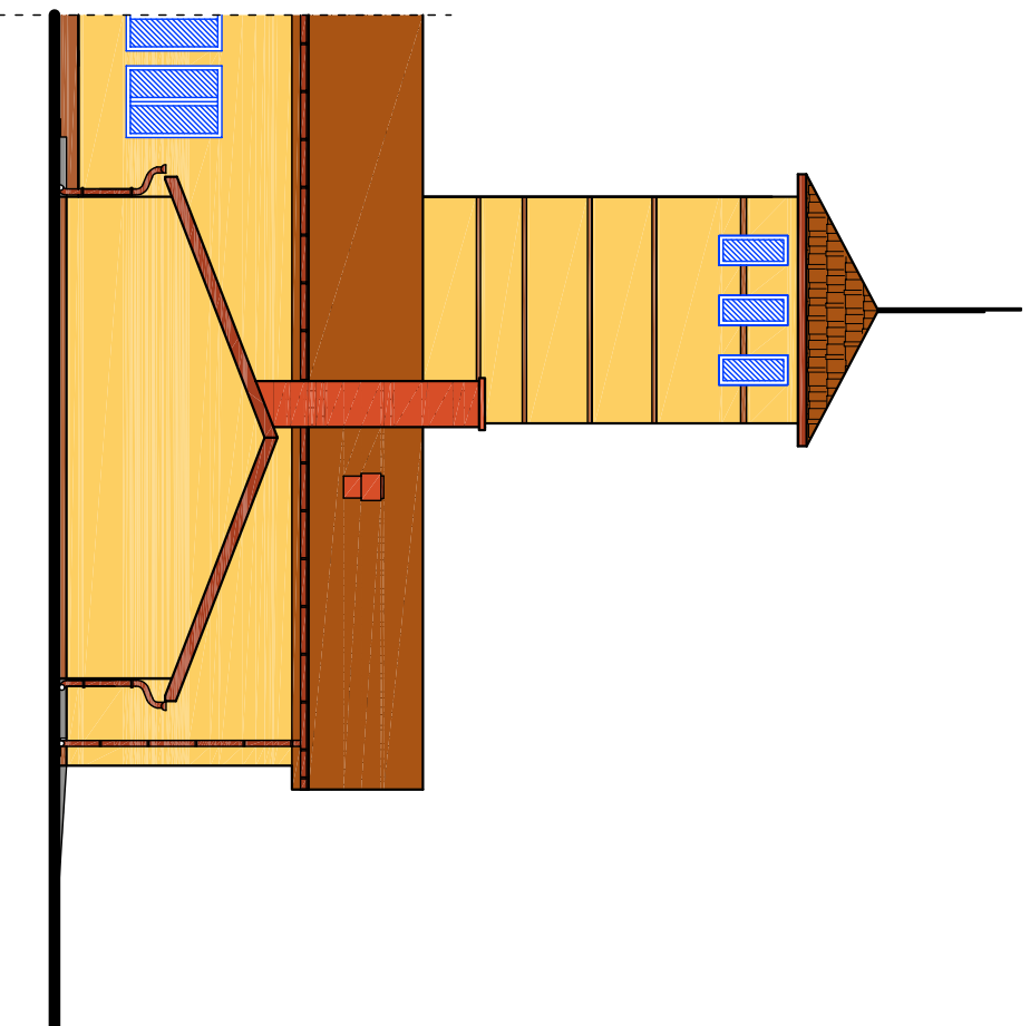
ELEWACJA ZACHODNIA 1:100
